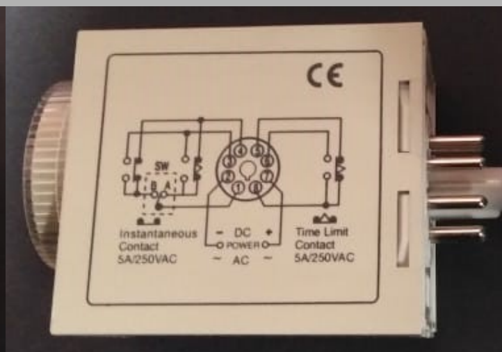
TEMPORIZADOR REF: H3-M1-220V
