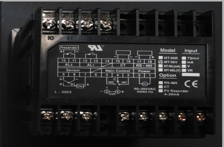
CONTROLADOR DE TEMPERATURA (PIROMETRO) REF: MT96-V
